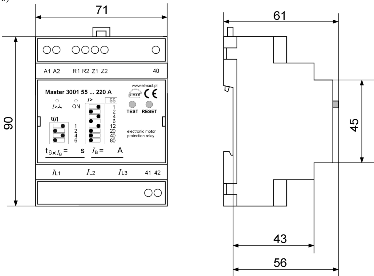
Rys. Nr 8. Wymiary zewnętrzne: a) sondy pomiarowej CR b) modułu operacyjnego
