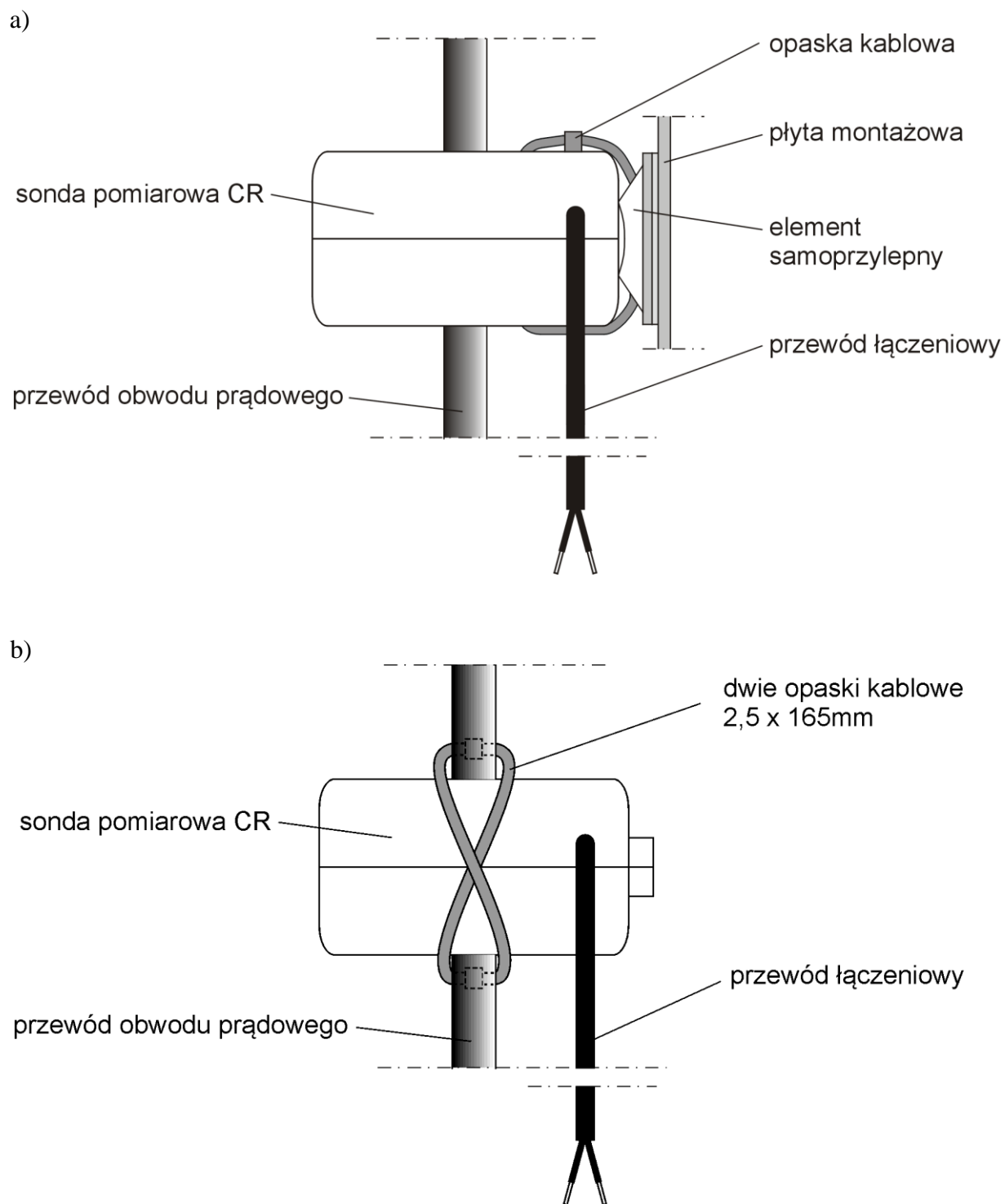
Rys. Nr 7. Mocowanie sond pomiarowych CR - widok z boku:
