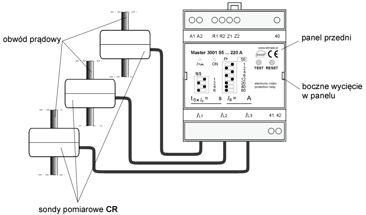
Rys. Nr 1. Zabezpieczenie Master 3001 – widok z przodu.
