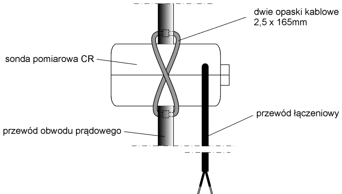
Rys. Nr 7. Mocowanie sond pomiarowych CR - widok z boku: a) na płycie, b) na przewodach obwodu prądowego.
