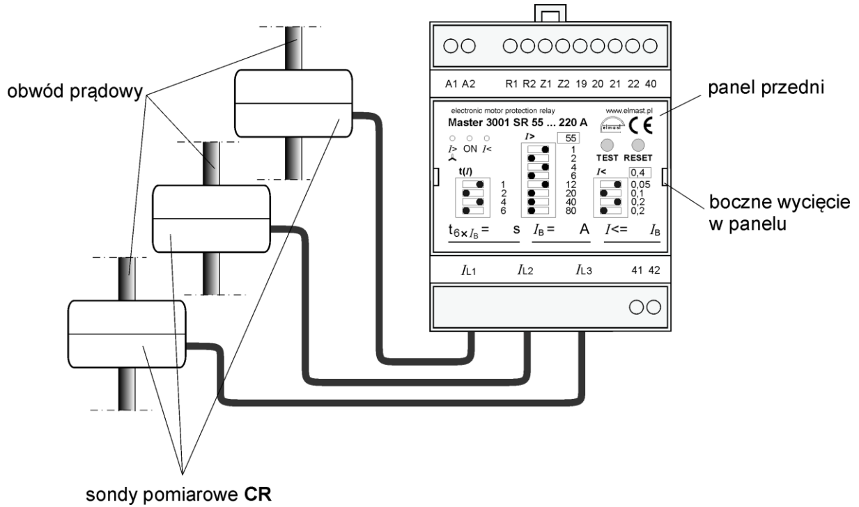
Rys. Nr 1. Zabezpieczenie Master 3001 SR – widok z przodu.
