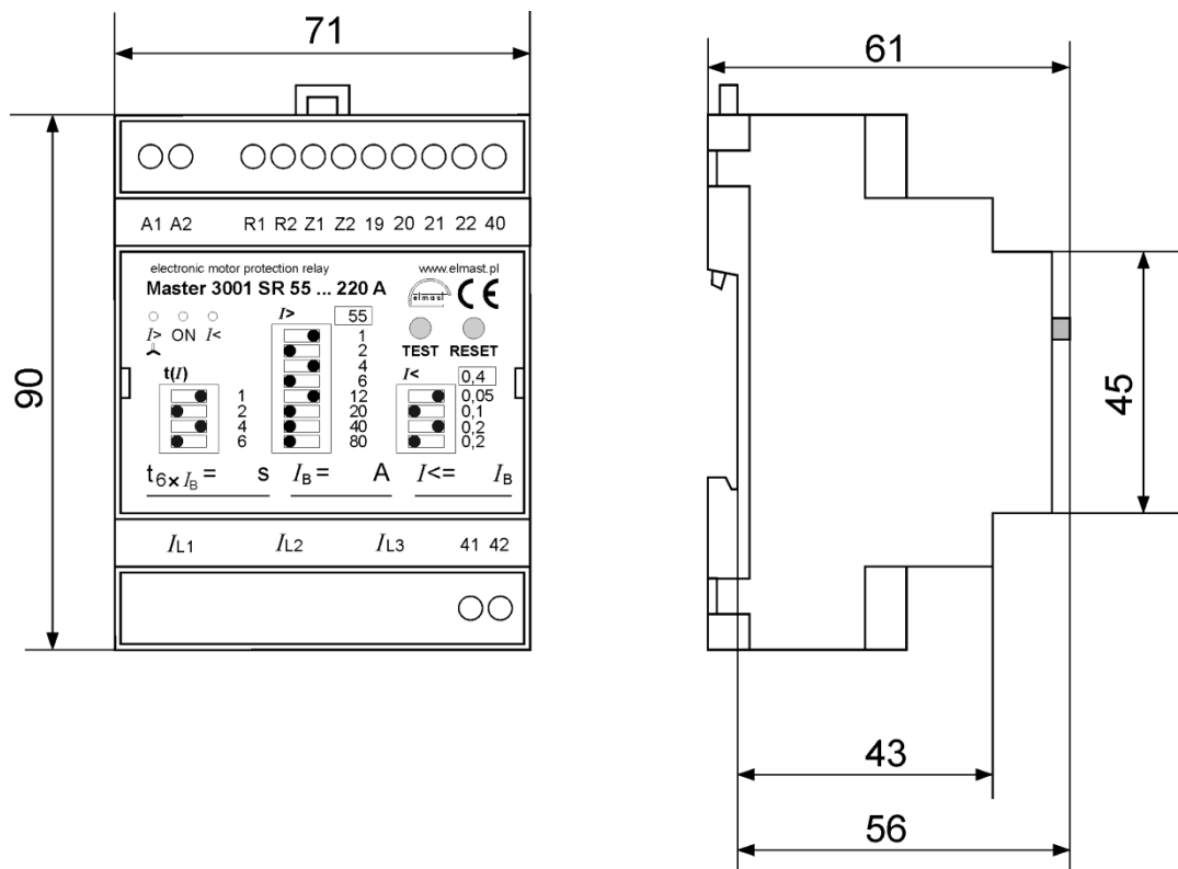
Rys. Nr 8. Wymiary zewnętrzne:
