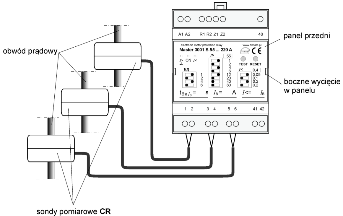
Rys. Nr 1. Zabezpieczenie Master 3001 S – widok z przodu.
