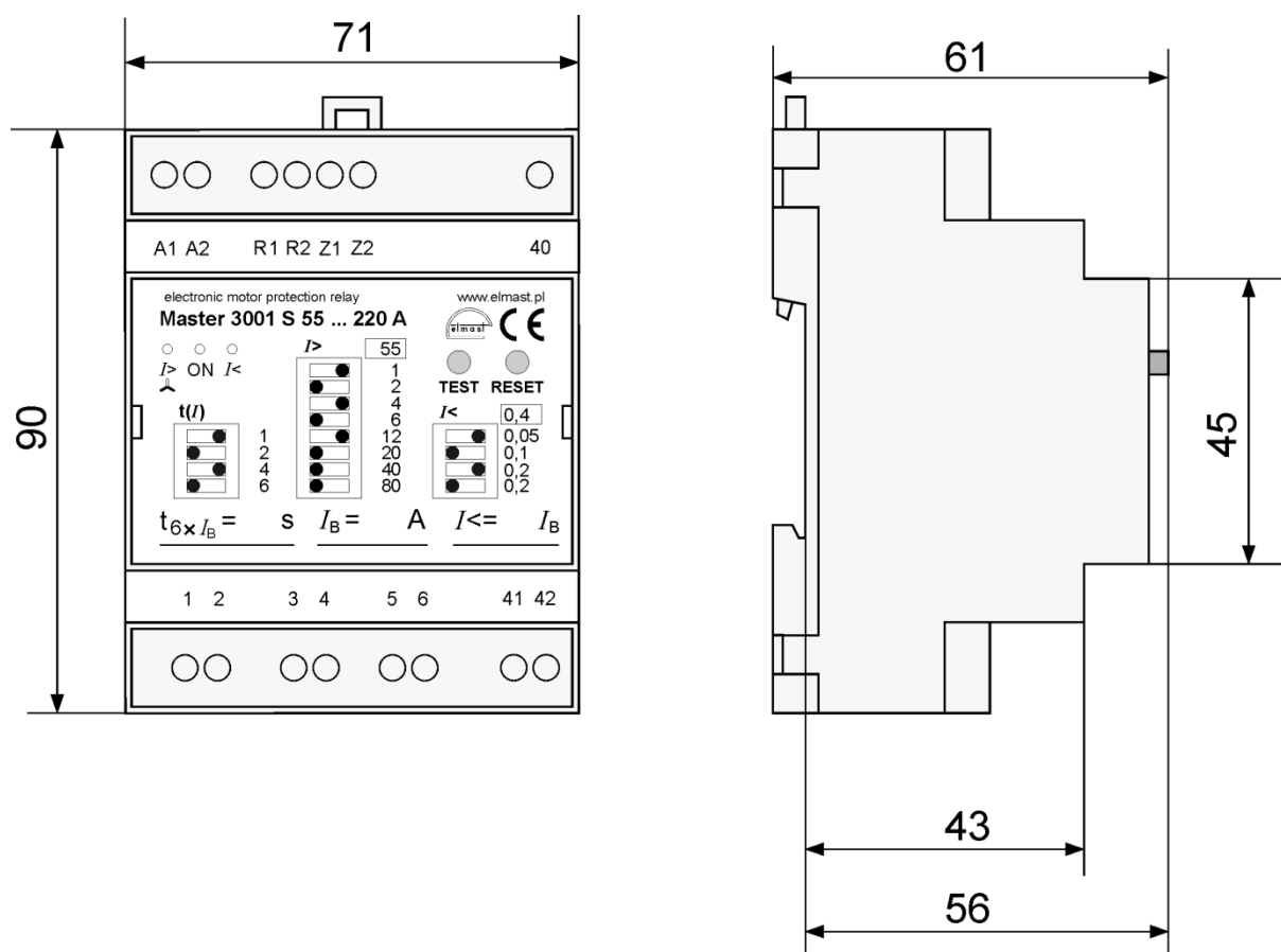
Rys. Nr 8. Wymiary zewnętrzne:
