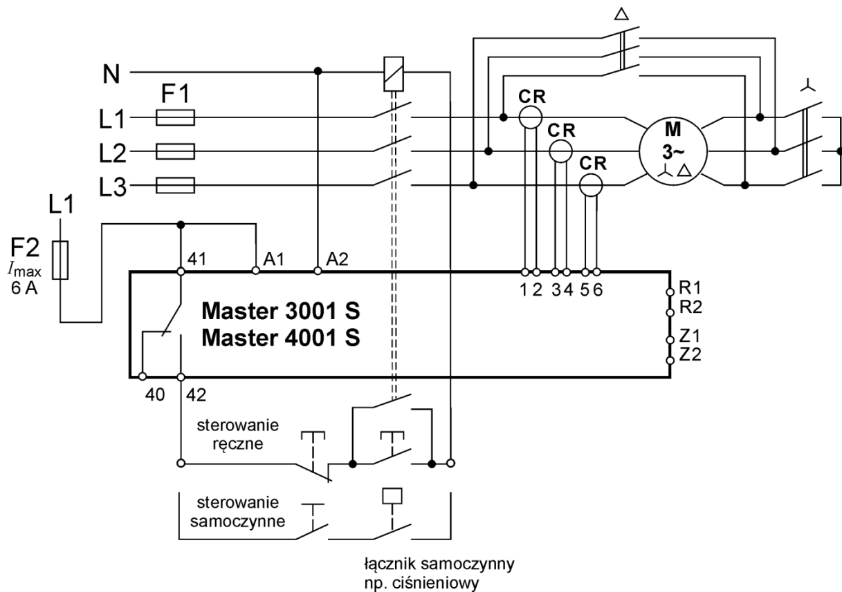
Rys. Nr 4. Schemat połączeń przy rozruchu \curvearrowright / \Delta I_B = 0,58 I_n ( I_B = 0,6 I_n )
