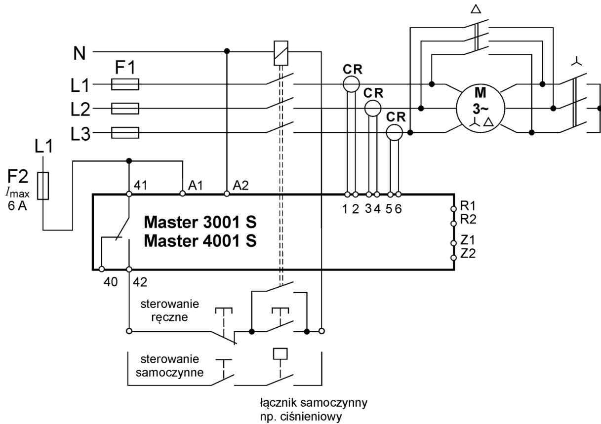
Rys. Nr 3. Schemat połączeń przy rozruchu \sphericalangle / \Delta I_B = I_n ( I_B = 1,05 I_n )
