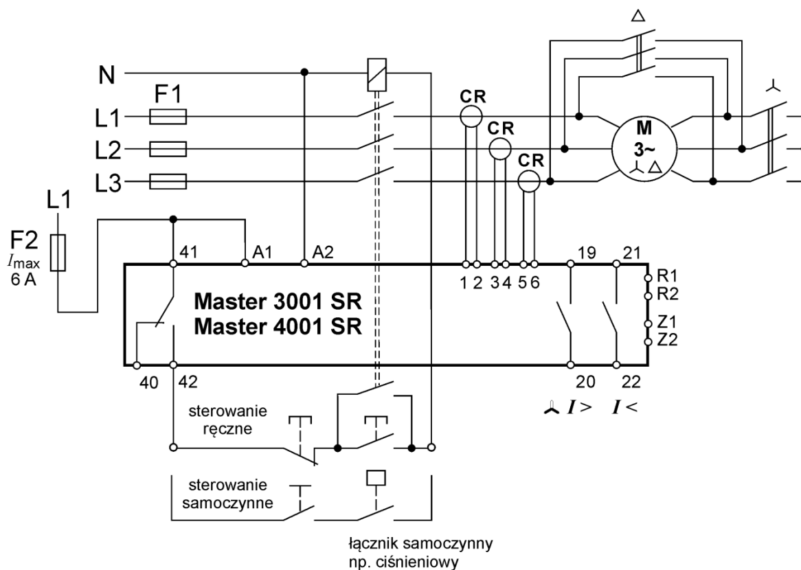
Rys. Nr 3. Schemat połączeń przy rozruchu \Delta / \Delta I_B = I_n ( I_B = 1,05 I_n )
