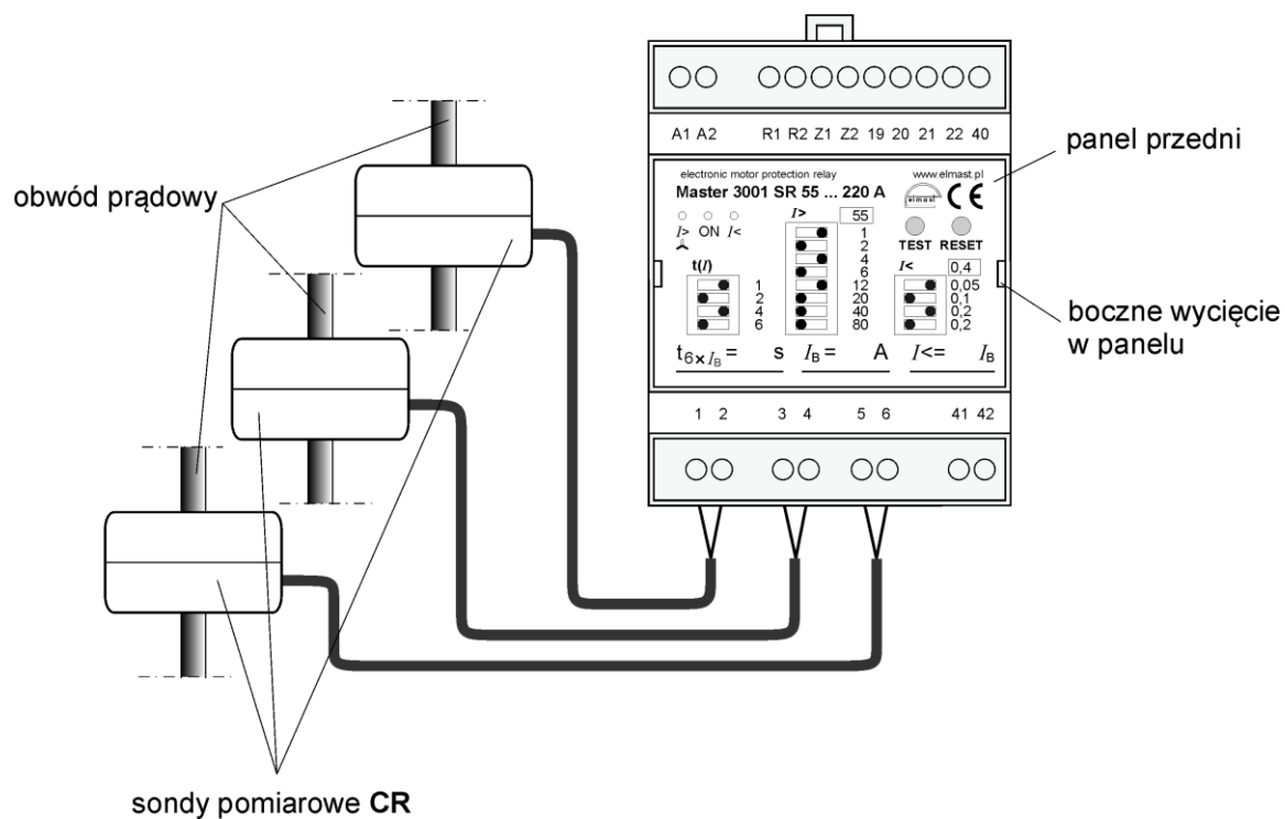
Rys. Nr 1. Zabezpieczenie Master 3001 SR – widok z przodu.
