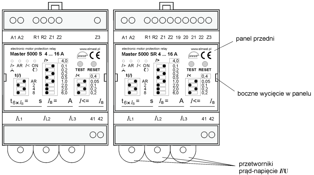
Rys. Nr 1. Zabezpieczenia Master 5000 S i Master 5000 SR - widok z przodu. Zakresy prądowe: 1,6 ... 6,3 A, 4 ... 16 A
