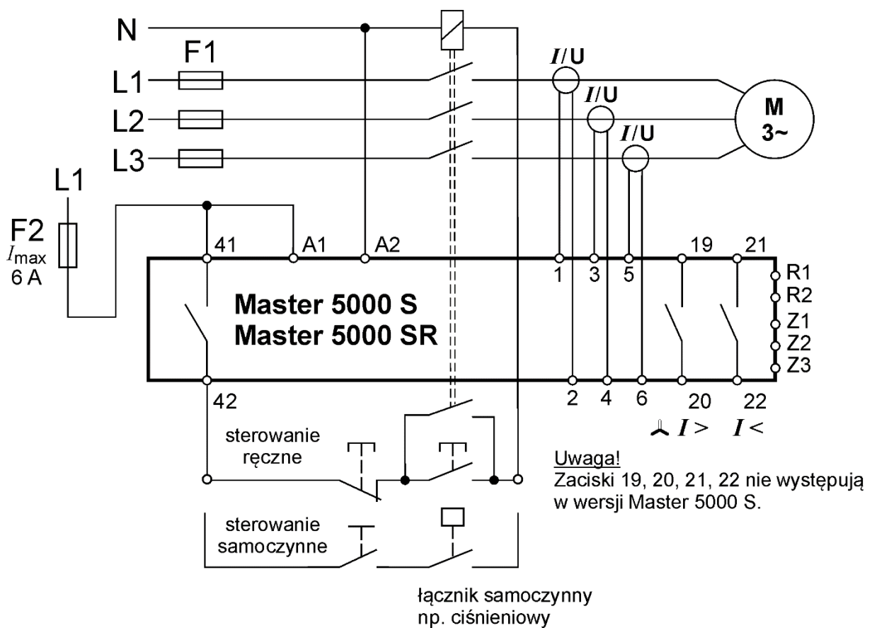
Rys. Nr 2a. Schemat połączeń przy rozruchu bezpośrednim I_B = I_n ( I_B = 1,05 I_n ) Zakresy prądowe: 10 ... 40 A, 16 ... 63 A, 55 ... 220 A
