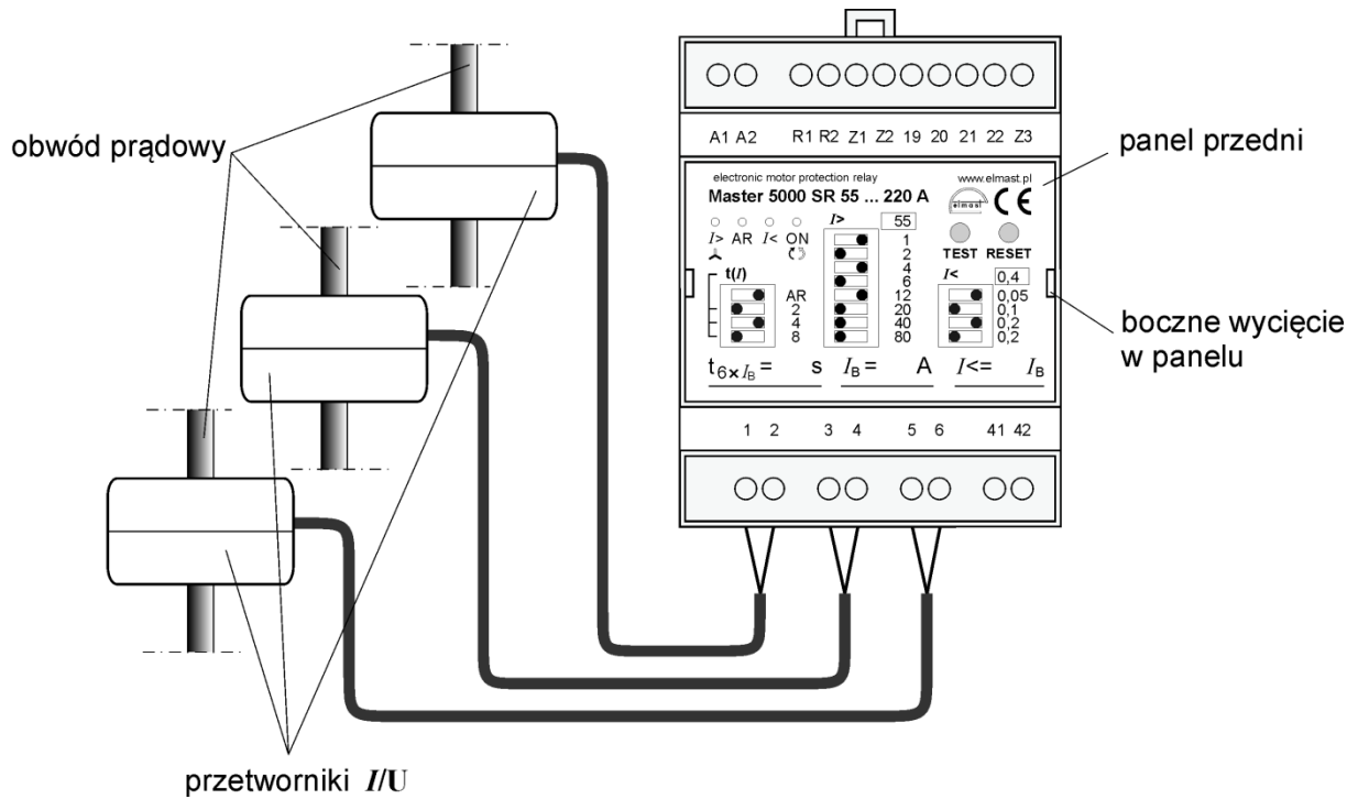
Rys. Nr 1a. Zabezpieczenie Master 5000 SR – widok z przodu. Zakresy prądowe: 10 ... 40 A, 16 ... 63 A, 55 ... 220 A
